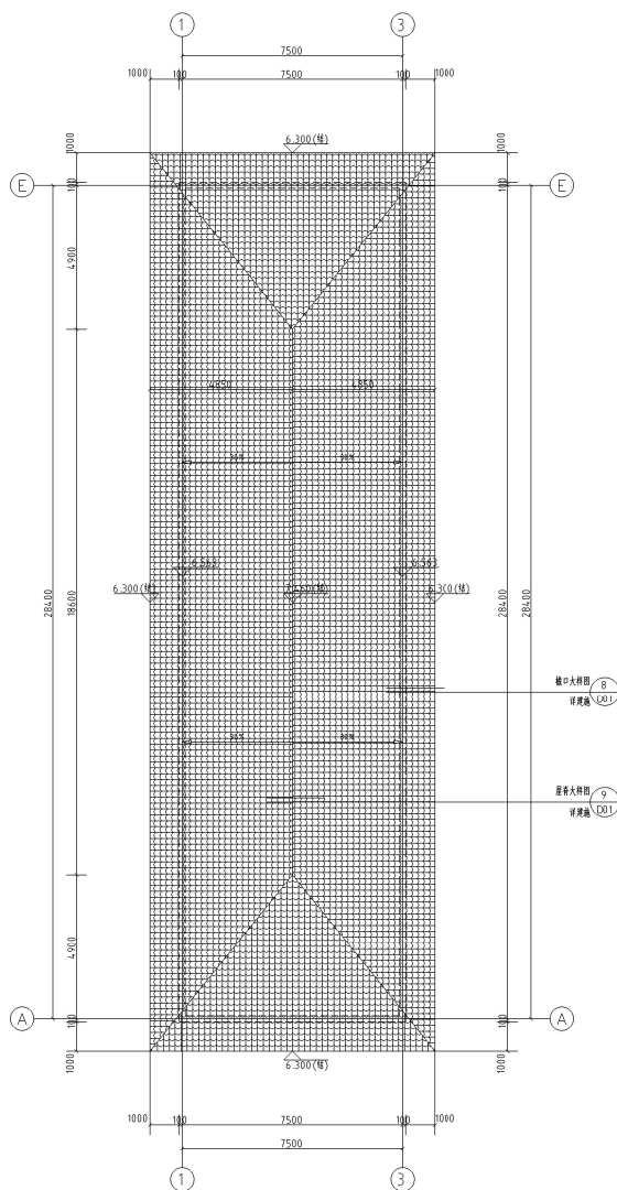
屋顶平面图 1:100
