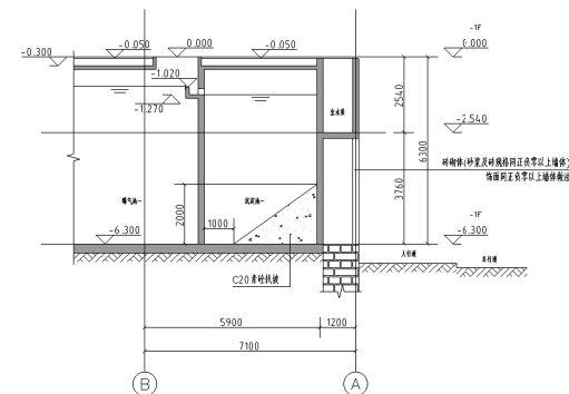
1-1 剖面图 1:100
